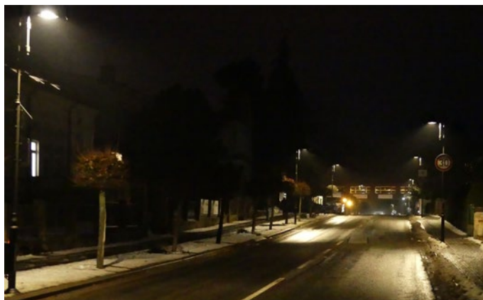
Soustava veřejného osvětlení I. etapa, realizace, investiční náklady 8 809 099 Kč
